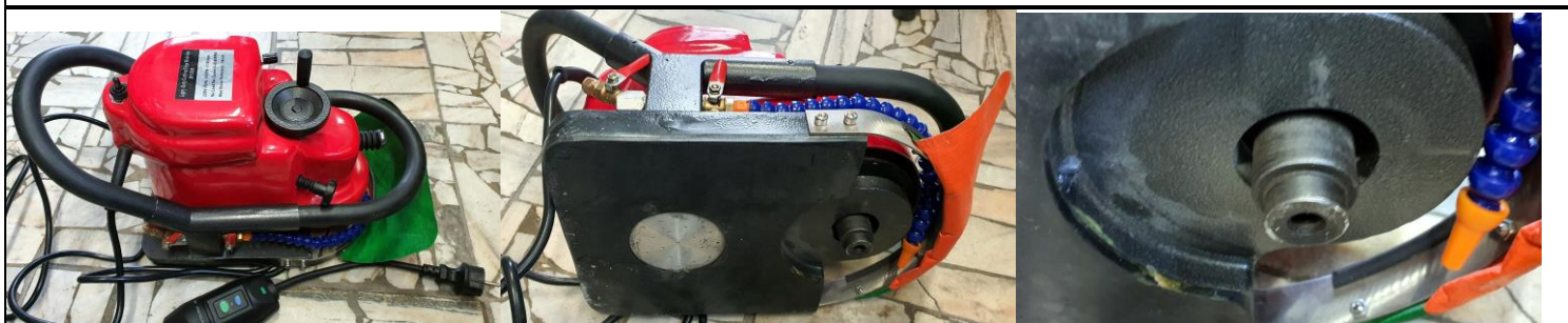
MY3009 jest profesjonalnym urządzeniem do obróbki profili bocznych płyt granitowych i marmurowych. Posiada własny napęd o mocy 2000W i prędkość 0-8500obr/min. Max grubość obrabianej płyty do 40mm. Posiada podajnik wody.
